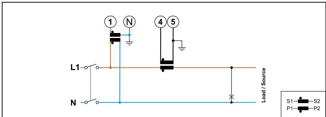
1 Faz, 2 iletken (VT/CT bağlantı soketi)
