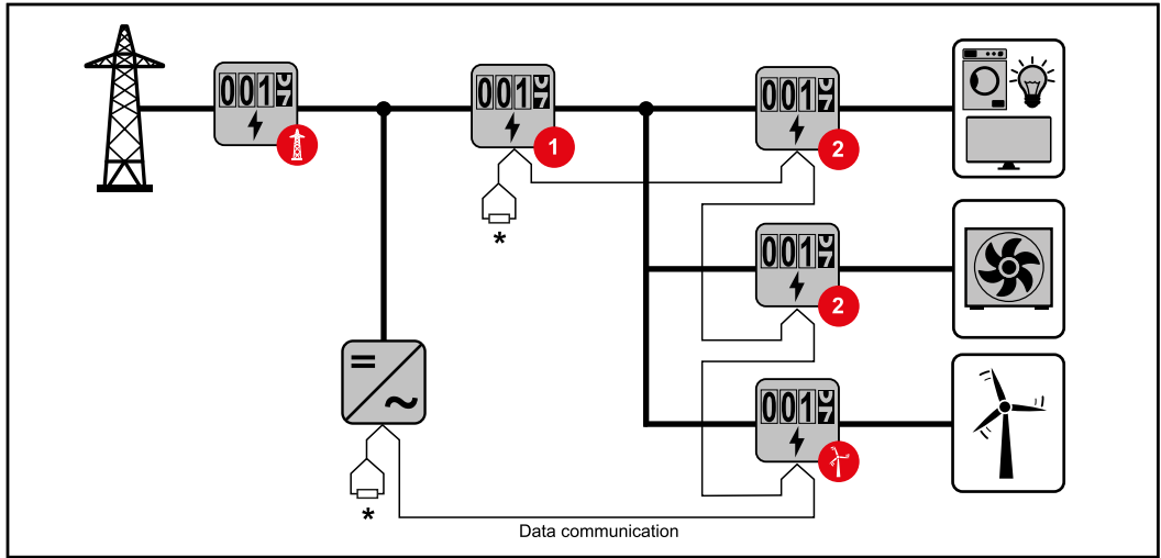
Tüketim bölümünde primer sayaçların konumu. Sonlandırma direnci R 120 \text{ Ohm}
