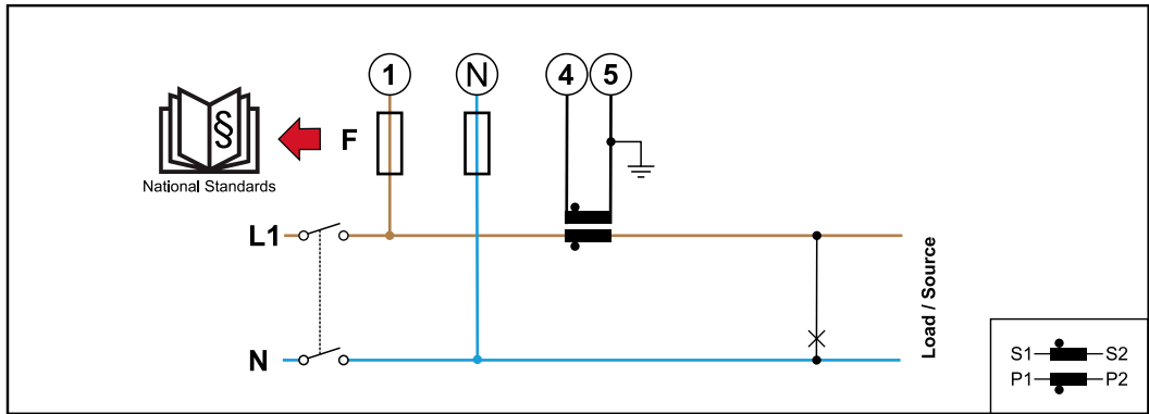
1 Faz, 2 iletken (CT bağlantı soketi)
