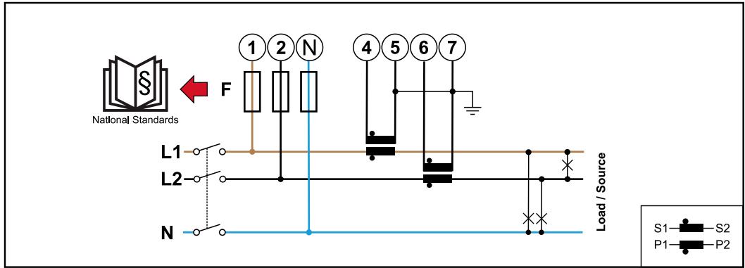
2 Faz, 3 iletken (CT baęlantı soketi)
