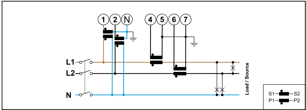
2 Faz, 3 iletken (VT/CT baęlantı soketi)
