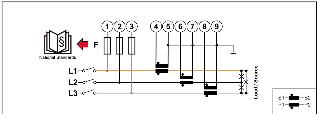
3 Faz, 3 iletken (CT baęlantı soketi)
