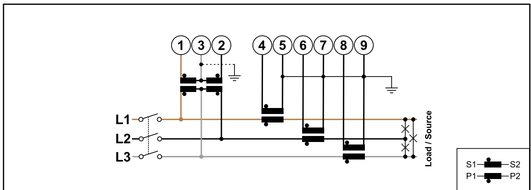
3 Faz, 3 iletken (VT/CT baęlantı soketi)
